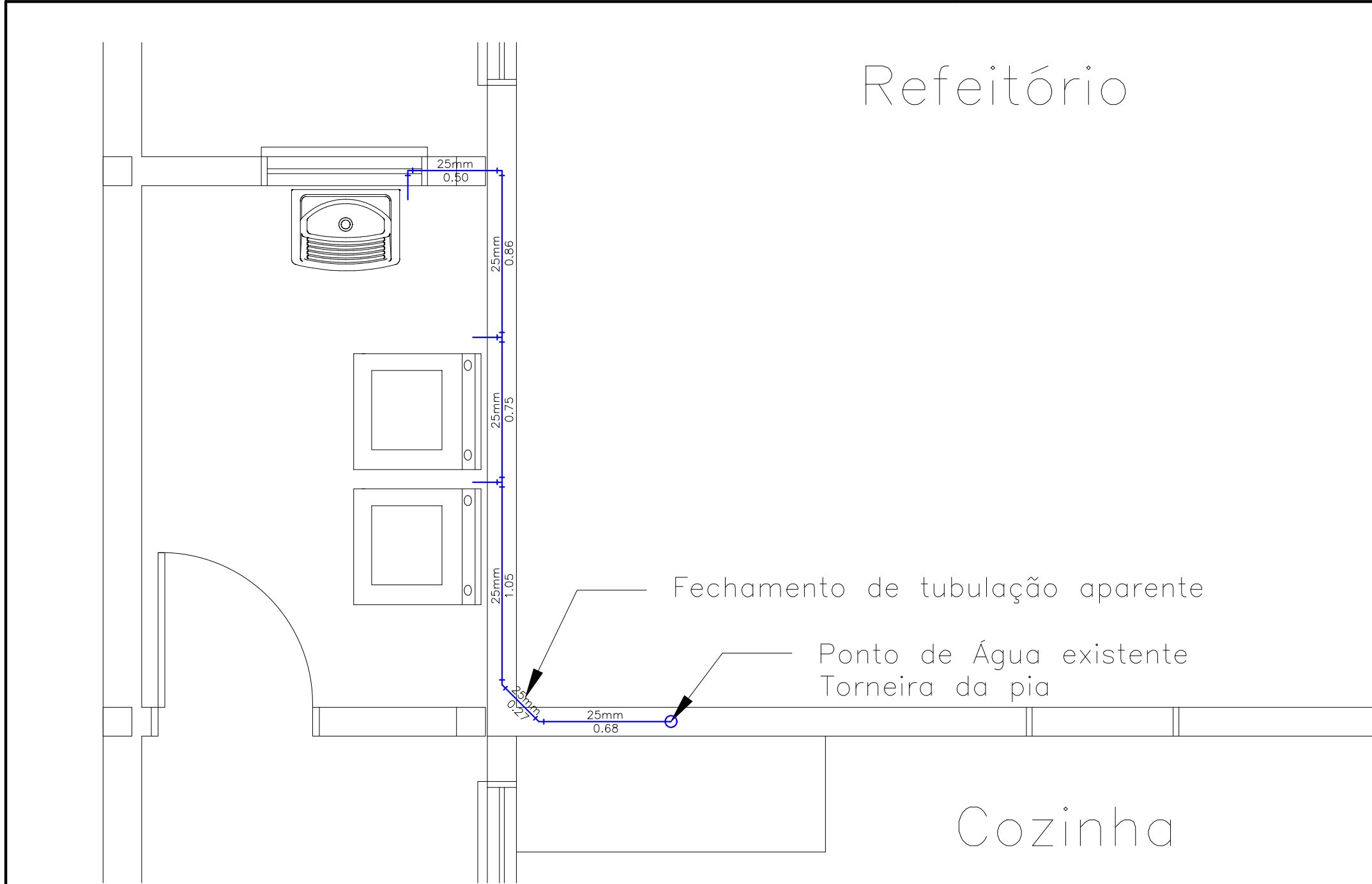
PLANTA BAIXA INSTALAÇÃO HIDRÁULICA COZINHA E SERVIÇOS ESCALA 1/25
