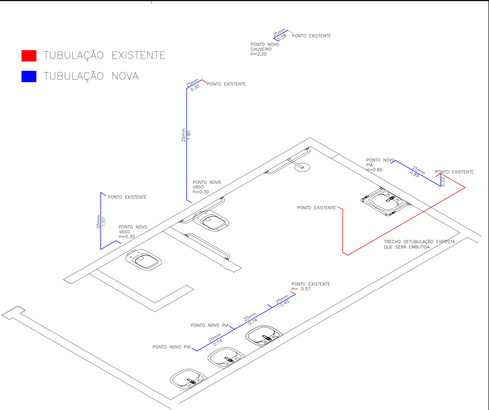
ISOMÉTRICO BANHEIRO ACESSÍVEL ESCALA 1/50
